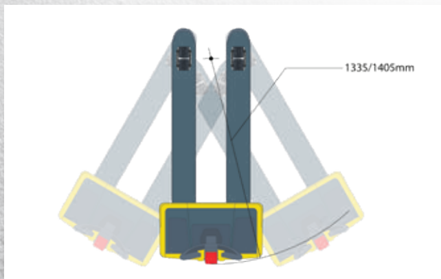
Transpaleta tipo MINI
